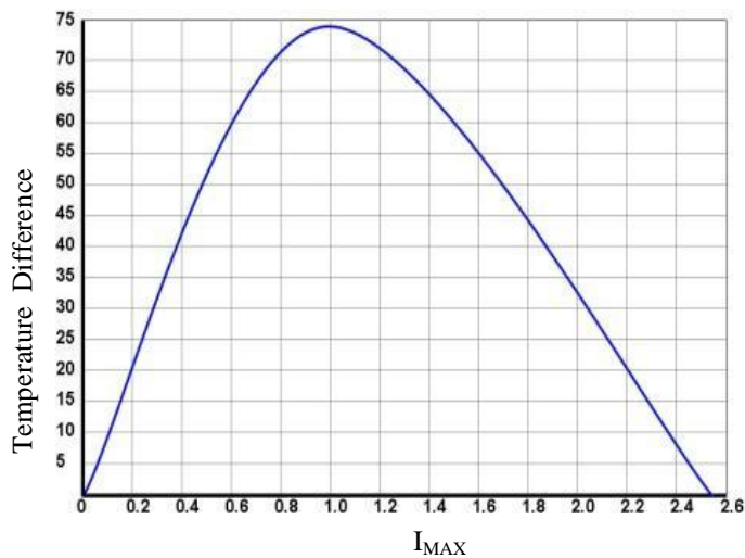
图 7. DT 与 I_{MAX} 的关系图
