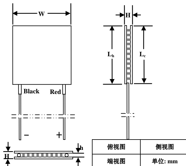
图11. 非密封ATE1-71的机械尺寸
