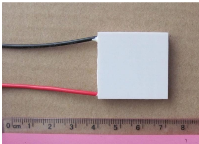
图 1.2 ATE1-71 的实体照片
