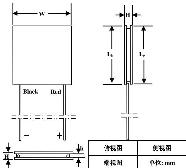
图 10. 密封ATE1-71的机械尺寸
