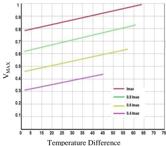
图 4. V_{MAX} 与DT的关系图
