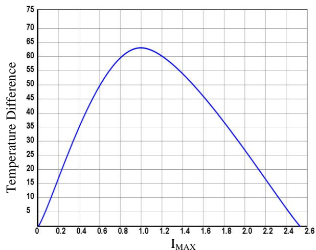
图3. DT与 I_{MAX} 的关系图
