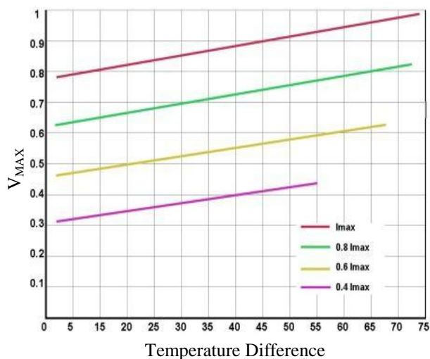
图 8. V_{MAX} 与 DT 的关系图
