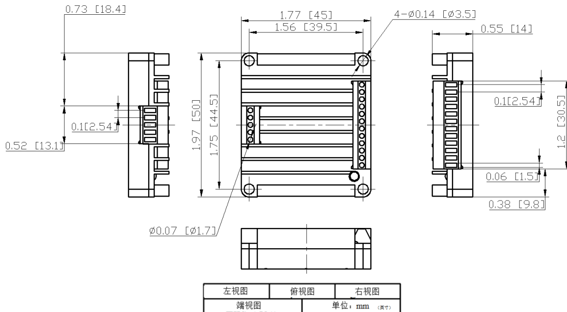
图 7. AQCL500MA410DF 的尺寸
