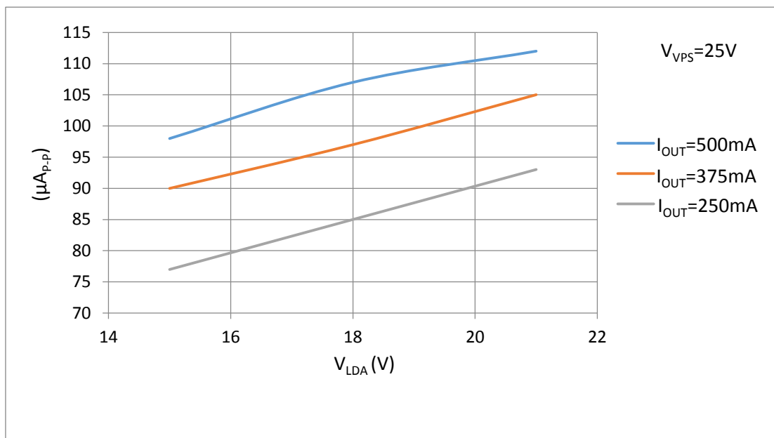
图 6. V_{LDA} vs. 输出电流噪声@0.1Hz~10Hz
