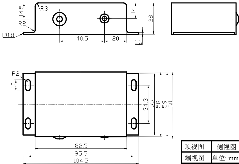
图12、HXHV24V7KV1MAW的尺寸
