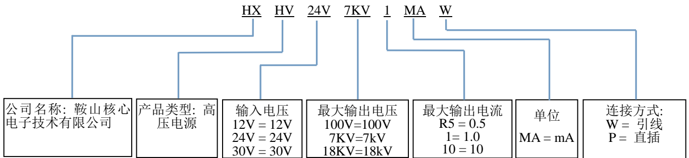
图 10、HXHV24V7KV1MAW 的命名说明
