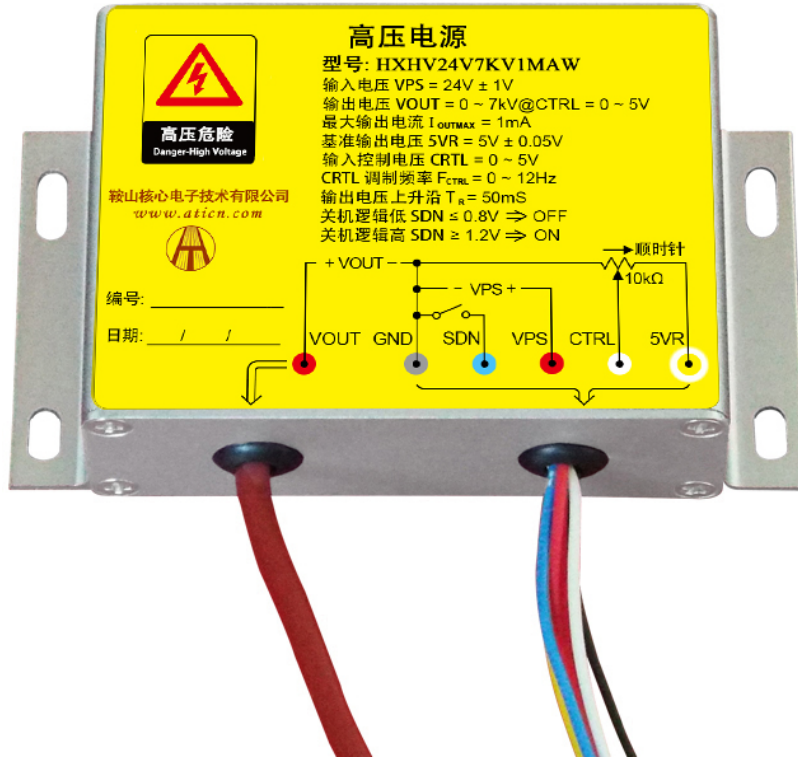
图 1、HXHV24V7KV1MAW 俯视图
