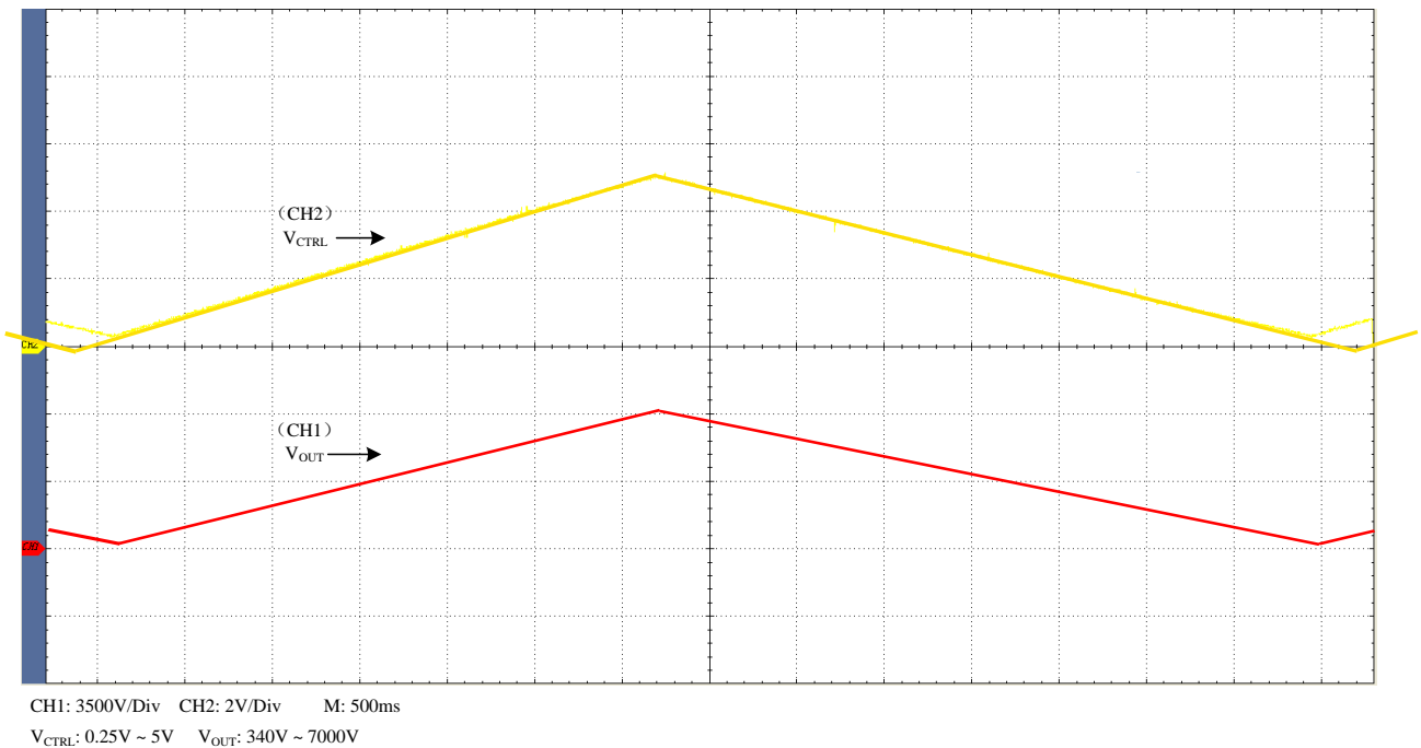
图3、三角波
