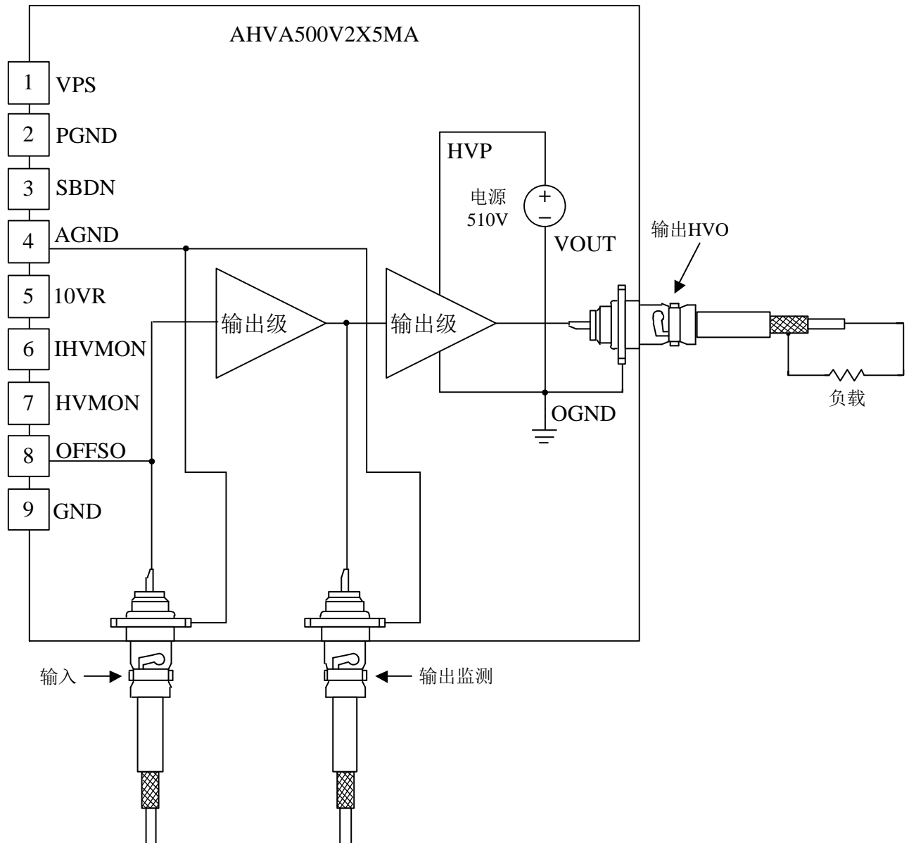
图 4、方框图和应用示意图
