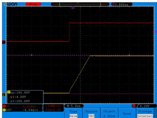
图 5、上升沿
