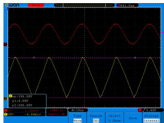
图 10、 f = 35kHz
