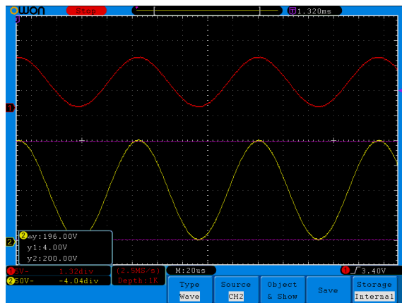
图 8、 f = 10kHz
