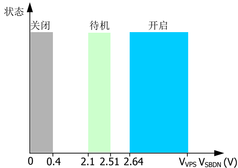
图 3、 V_{\text{SBDN}} VS. 放大器状态
