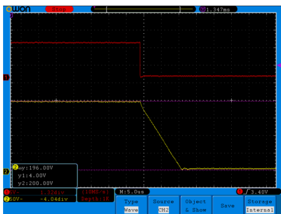
图 6、下降沿
