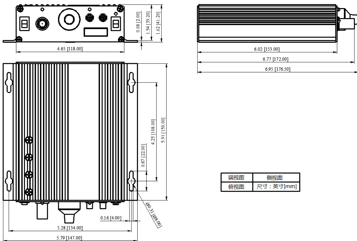
图12、AHVA2KV2X5MA的尺寸图
