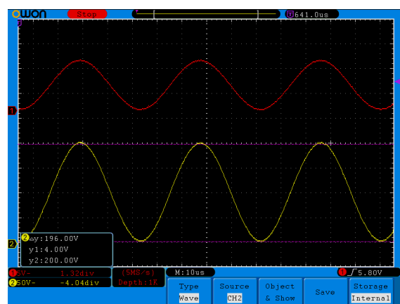
图 9、 f = 20kHz
