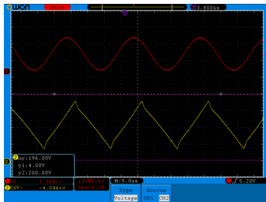
图 11. f=50\text{kHz}
