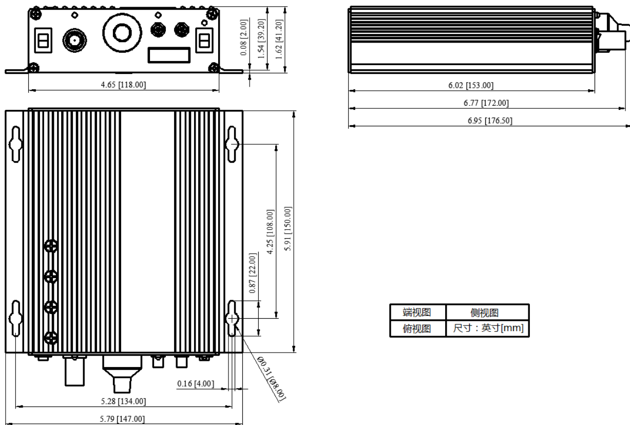
图11、AHVA250V2X20MA的尺寸图
