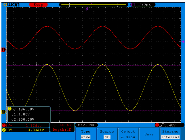
图 5、 f = 100\text{Hz}
