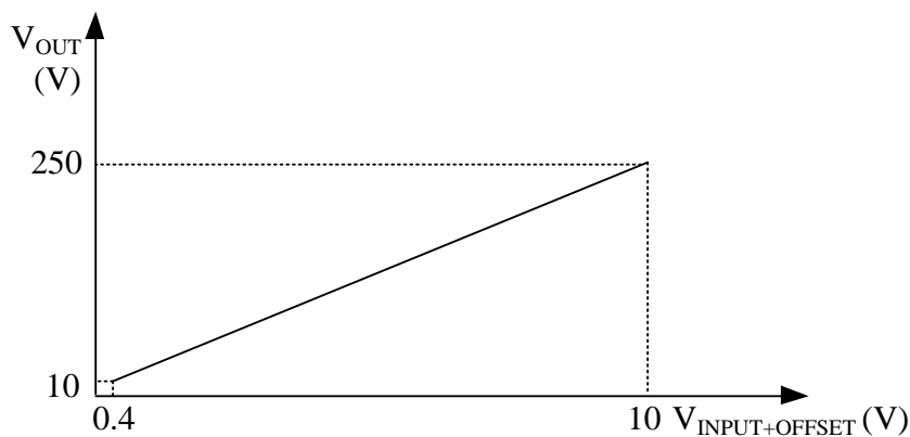
图 2、 V_{OUT} vs. V_{VIN}
