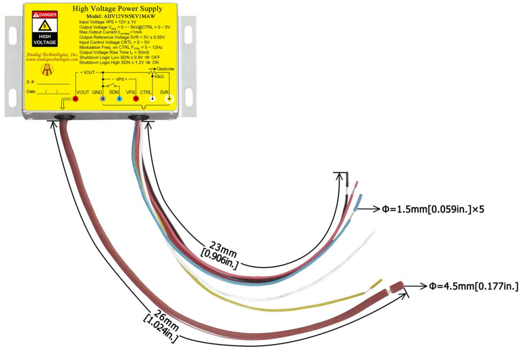
图11、AHV12VN5KV1MAW的导线
