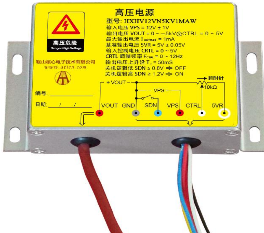
图 1、AHV12VN5KV1MAW 俯视图
