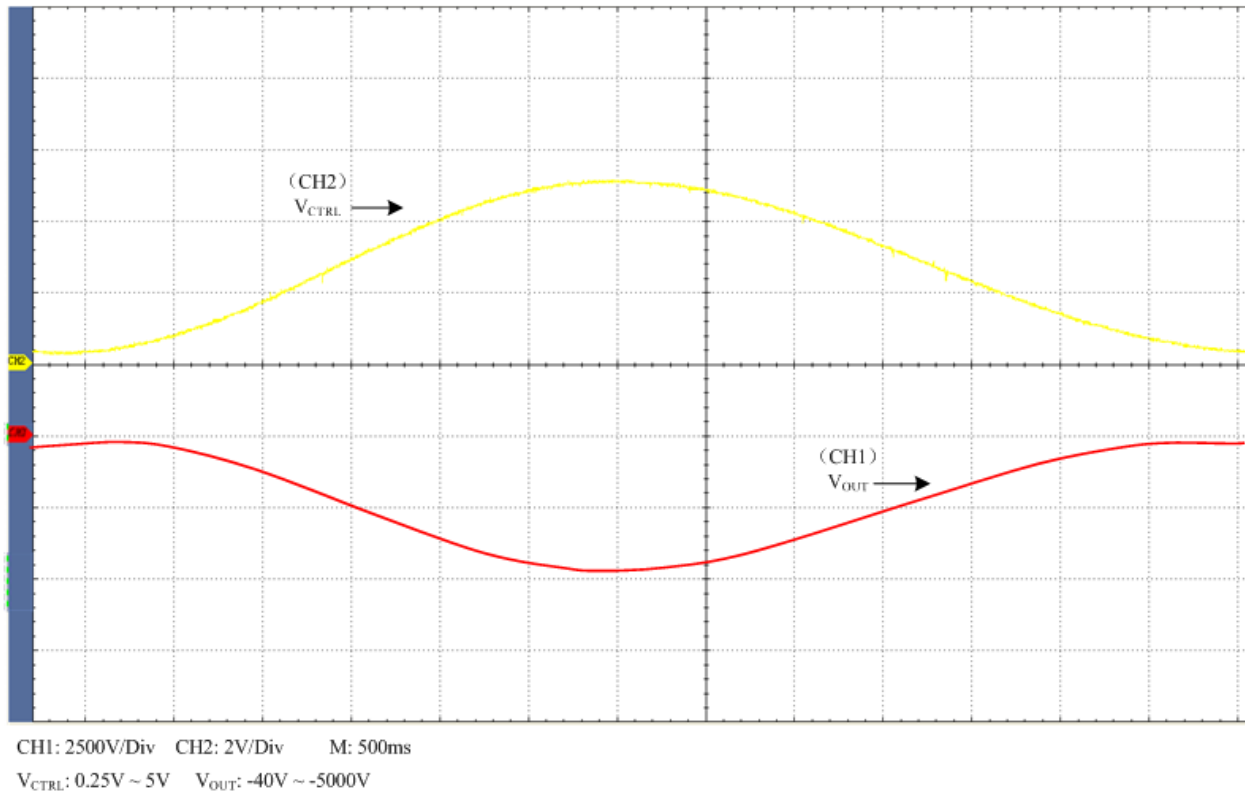
图4、正弦波
