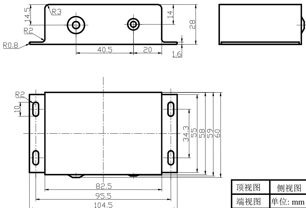
图12、AHV12VN5KV1MAW的尺寸
