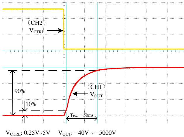
图6、上升沿时间
