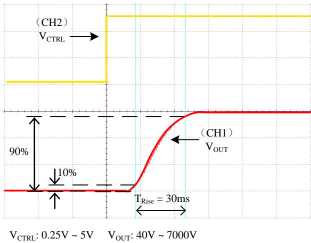
图6、上升沿时间
