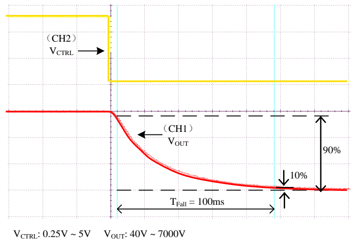
图7、下降沿时间
