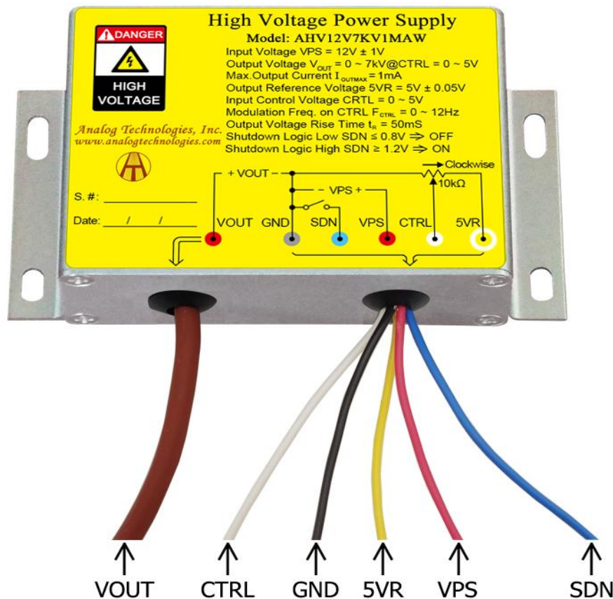
图 1、AHV12V6KV3MAW 俯视图
