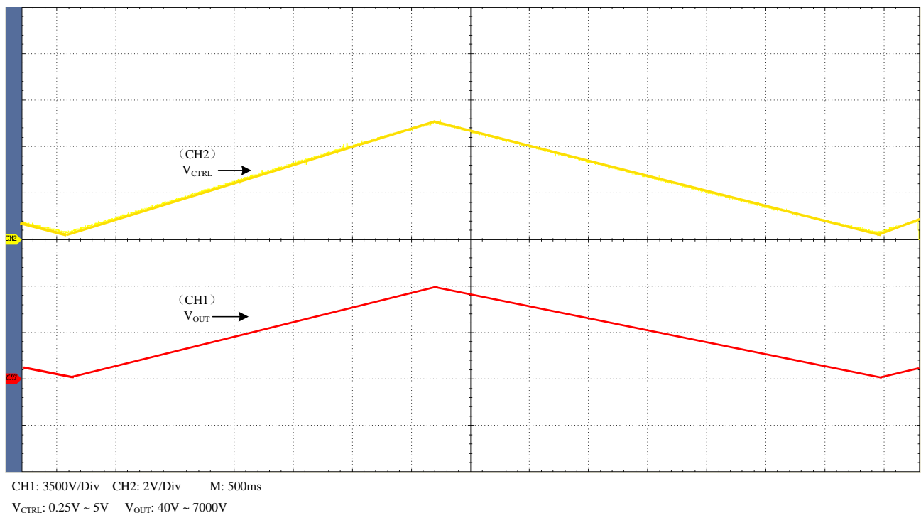
图3、三角波
