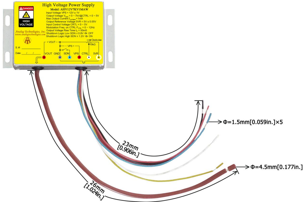
图11、AHV12V6KV3MAW的导线
