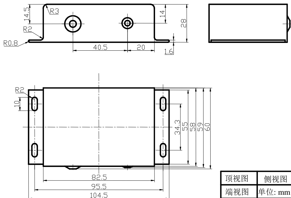
图12、AHV12V6KV3MAW的尺寸
